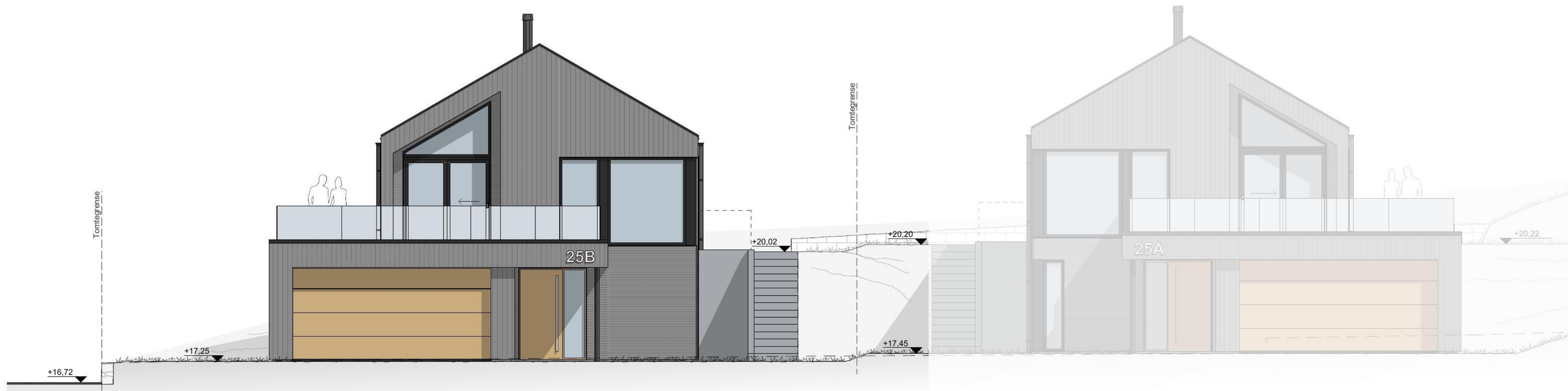
Fasade mot SØR-ØST bolig B
